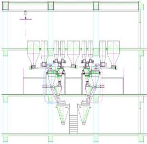
Obr.2.: Celé technologické schéma linky
