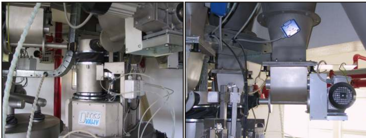
Obr.5.: Plnění do vah šnekovými podavači
